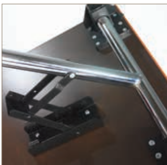
Klappmechanismus Gefederte Clips halten die Tischbeine in Position, wenn geklappt
